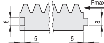
ZCR-A (M = 4)
