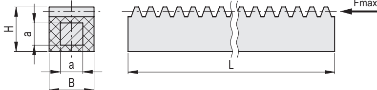
ZCR-A (M ≤ 3)
